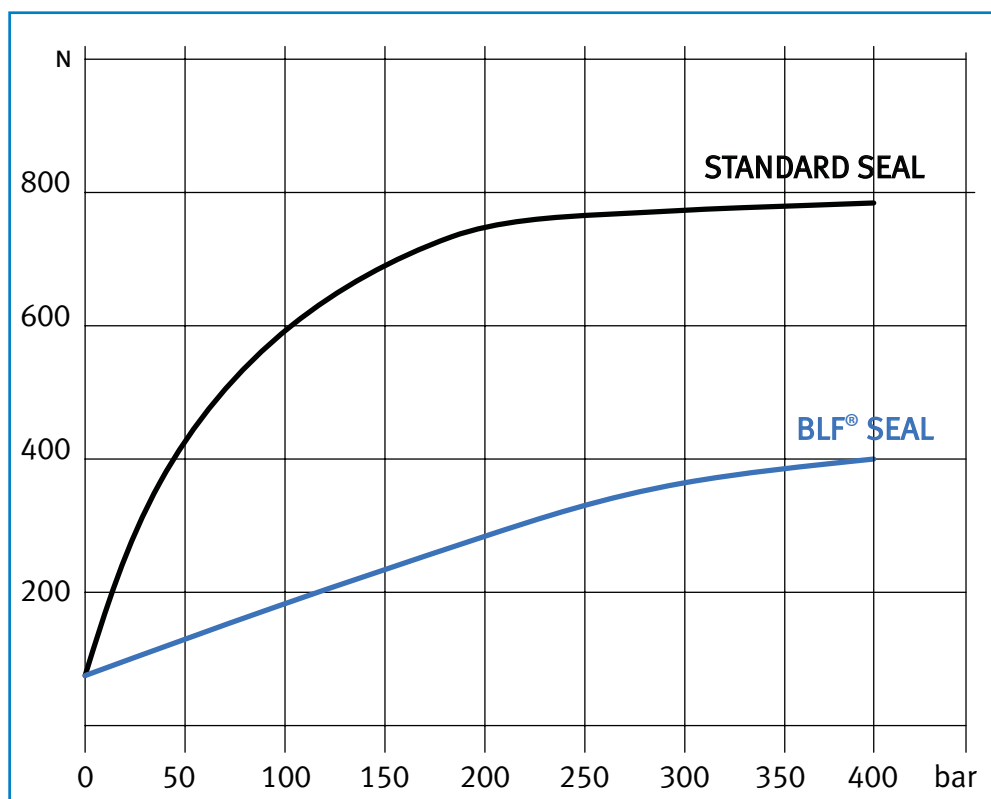
Fig. 31 PRESSIONE/ATTRITO - Pic.31: PRESSURE/OPERATING FRICTION
